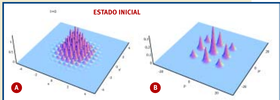
Figura 5. A experiência de Florença (Itália), semelhante à da figura 3, mas com átomos ‘deslocalizados’ que podem ocupar um grande número de regiões da armadilha, separadas por barreiras (a). Em (b), a distribuição de momentos \rho(p, p' = p) mostra três máximos, além de outros em regiões com p' \neq p . O estado final exhibe três grupos separados de átomos (c), como observado experimentalmente (d)
