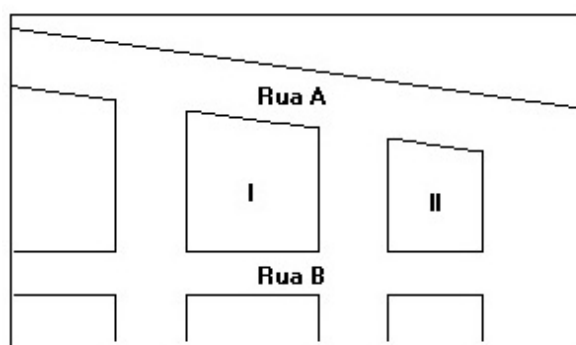
Figura 52 – Aplicação 5 contextualizada do Teorema de Tales para segmentos proporcionais. Fonte: UNIRIO
