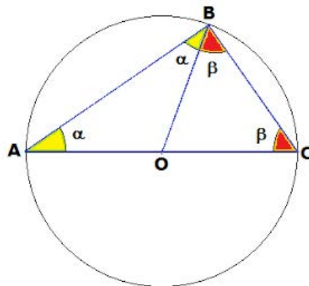
Figura 2 – Teorema de Tales no Círculo.
