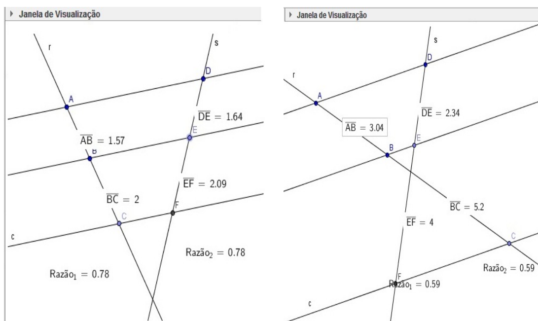
Figura 47 – Verificando as Proporções do Teorema de Tales 2.2.
