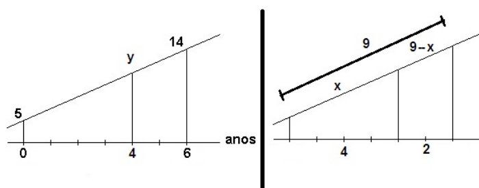
Figura 56 – Solução do problema de 4.2.2.2.
