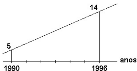
Figura 49 – Aplicação 2 contextualizada do Teorema de Tales para segmentos proporcionais. Fonte: Universidade Estadual de Londrina.
