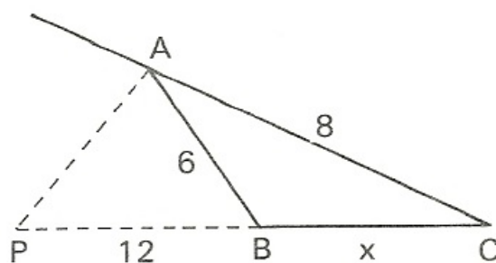
Figura 18 – Exemplificando o Teorema 2.5
