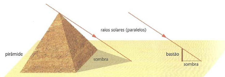
Figura 22 – Cálculo da altura da Pirâmide por meio de sua sombra. Fonte: (CENTURION; JAKUBOVIC, 2012)
