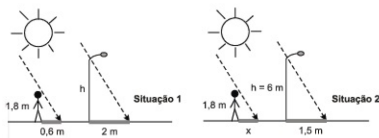
Figura 37 – Aplicando o Teorema de Tales em atividade 1 de Proporção. Fonte: www.sprweb.com.br em 25 de julho de 2013.
