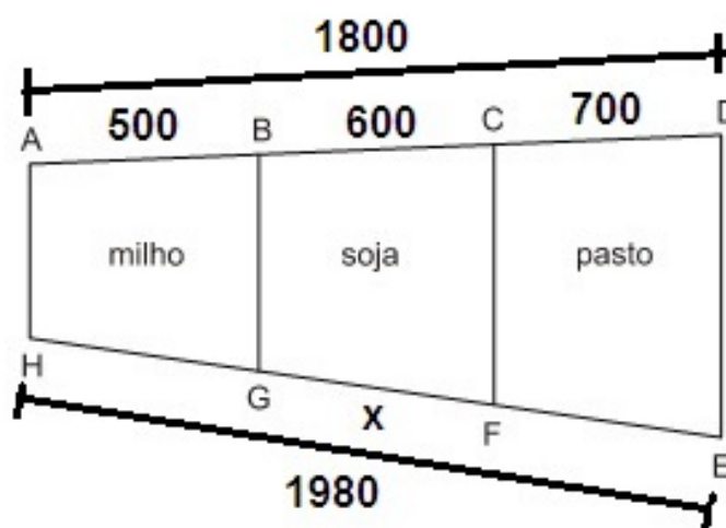
Figura 57 – Solução do problema de 4.2.2.4
