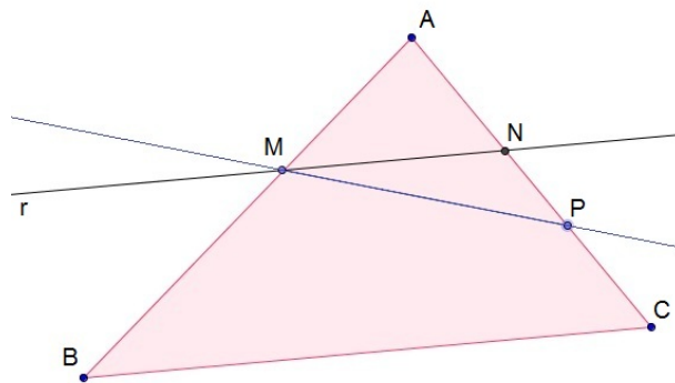
Figura 11 – Demonstrando o Teorema 2.3 por contraposição
