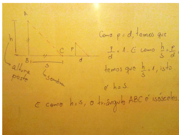
Figura 28 – Demonstração entre a altura do poste e a sombra e a relação no triângulo isósceles.
