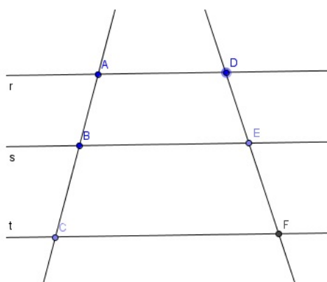
Figura 35 – Aplicando o Teorema de Tales 2.2.
