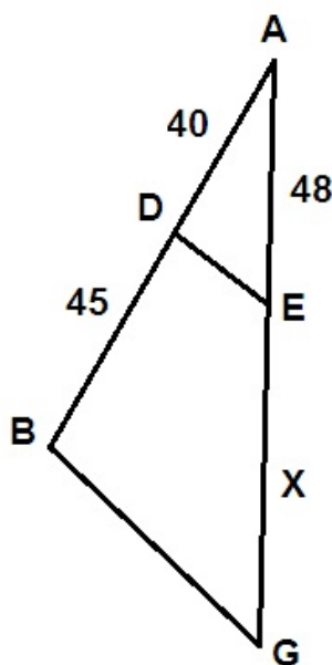
Figura 59 – Solução do problema de 4.2.2.6.
