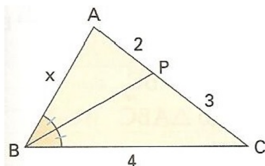
Figura 15 – Exemplificando o Teorema 2.4.
