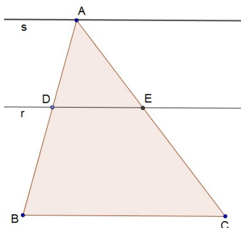
Figura 12 – Demonstrando o Teorema 2.3 usando proporções.
