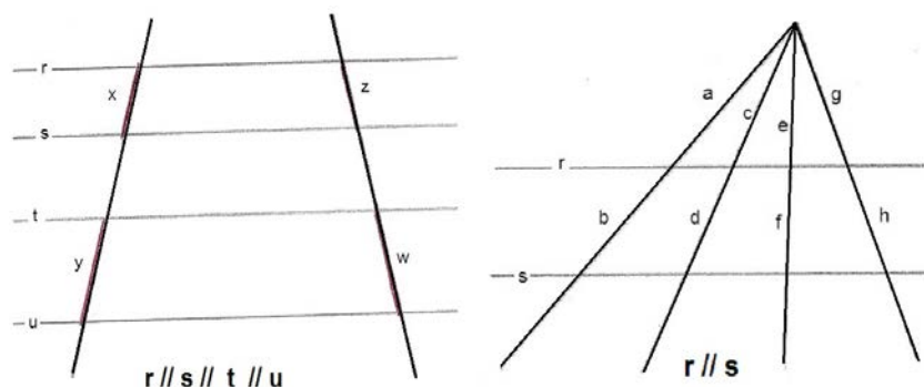
(a) Teorema de Tales na Itália e Espanha (b) Teorema de Tales na Alemanha
