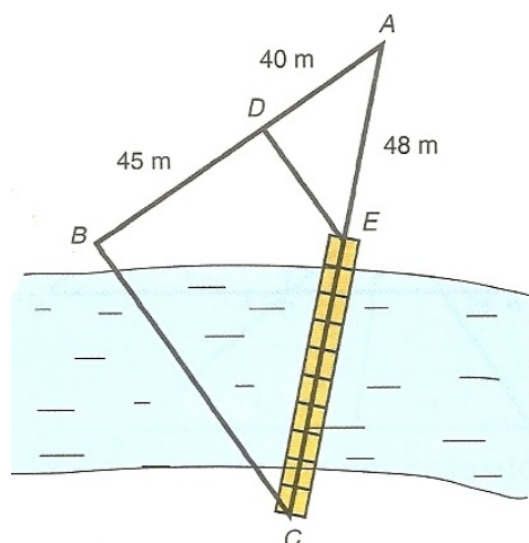
Figura 53 – Aplicação 6 contextualizada do Teorema de Tales para segmentos proporcionais. Fonte: (BIANCHINI, 2013).
