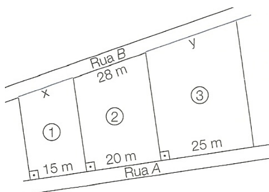
Figura 54 – Aplicação 7 contextualizada do Teorema de Tales para segmentos proporcionais. Fonte: (IEZZI; DOLCE; MACHADO, 2009).
