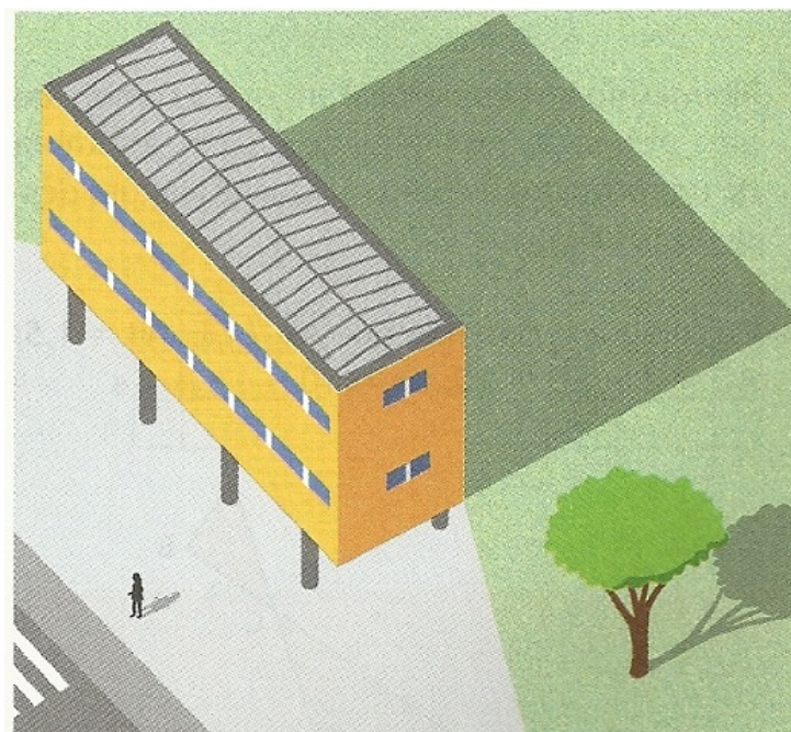
Figura 29 – Cálculo da altura de um prédio, usando medição da sombra. Fonte: (CENTURION; JAKUBOVIC, 2012)
