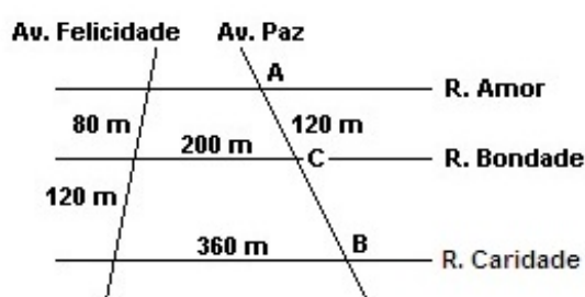
Figura 48 – Aplicação 1 contextualizada do Teorema de Tales para segmentos proporcionais. Fonte: Colégio Pedro II.
