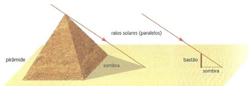
Figura 3 – Retas paralelas.
