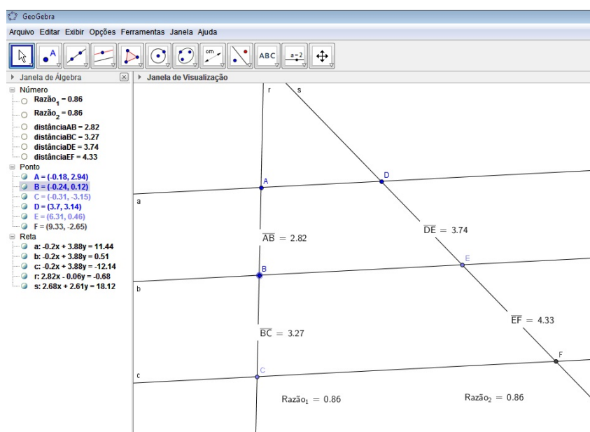
Figura 46 – Verificando o Teorema 2.2 no GeoGebra.
