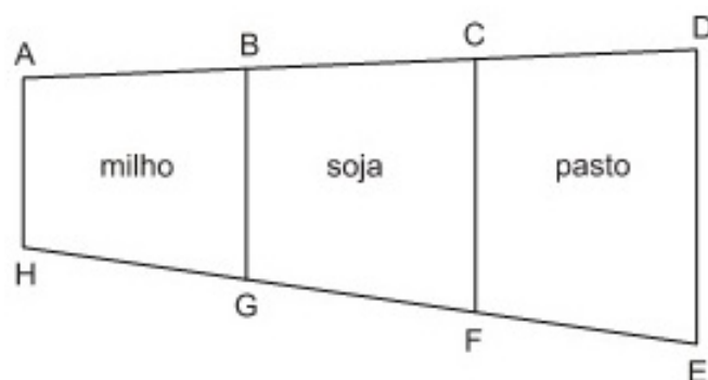
Figura 51 – Aplicação 4 contextualizada do Teorema de Tales para segmentos proporcionais. Fonte: Colégio Pedro II
