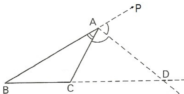
Figura 16 – O Teorema 2.5.
