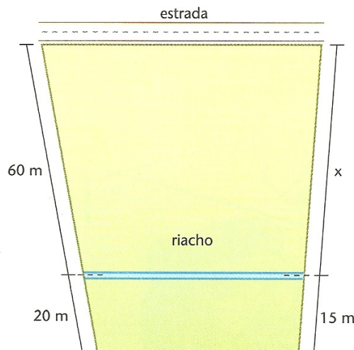
Figura 7 – Terreno na forma de trapézio, exemplificando o Teorema 2.2.
