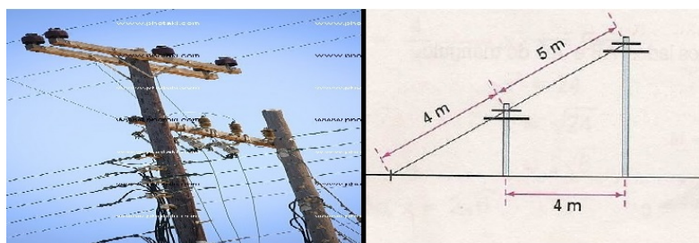
Figura 36 – Aplicando o teorema de Tales em atividade 1 de Proporção. Fonte: (JÚNIOR; CASTRUCCI, 2009).
