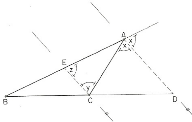
Figura 17 – Demonstrando o Teorema 2.5.
