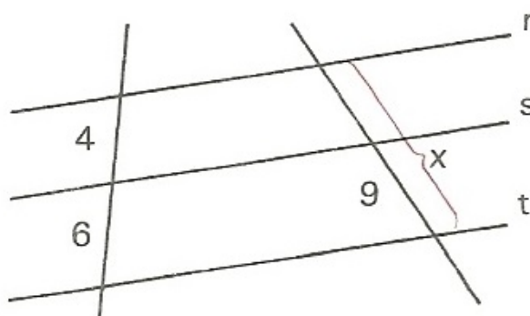
Figura 40 – Aplicando o Teorema de Tales em atividade 5 através de feixe de retas paralelas. Fonte: (DOLCE; POMPEO, 2001).
