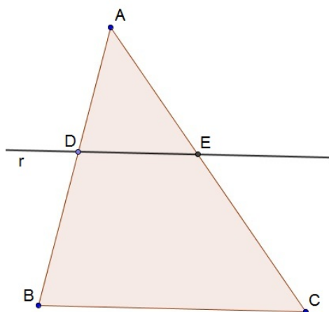
Figura 9 – O Teorema de Tales 2.3 (No Triângulo).
