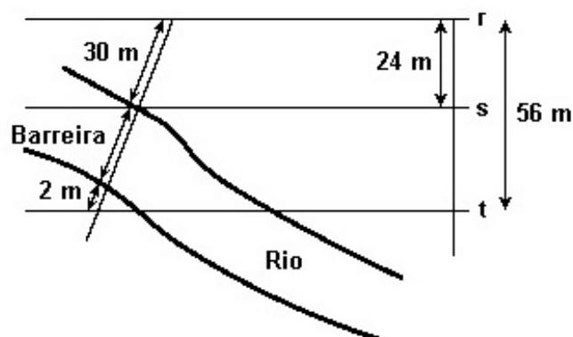
Figura 38 – Aplicando o Teorema de Tales em atividade 3 de Proporção. Fonte: Vestibular da UFSM
