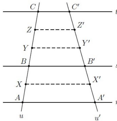
Figura 6 – Demonstrando o Teorema 2.2.
