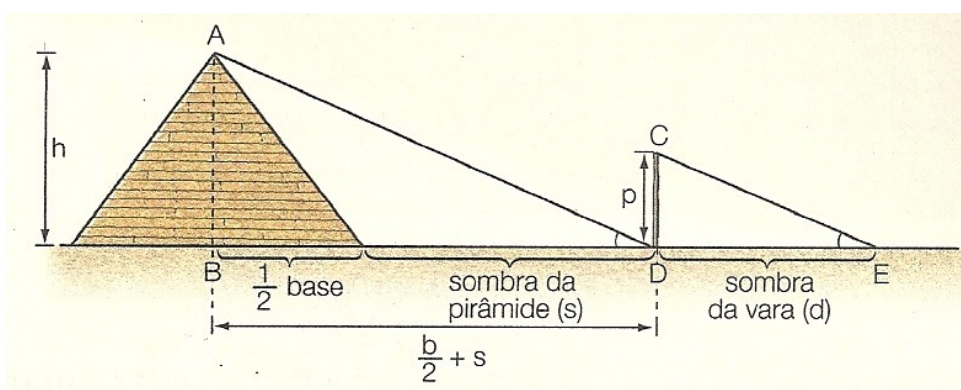
Figura 24 – Fonte (IEZZI; DOLCE; MACHADO, 2009).
