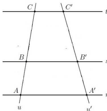
Figura 5 – O Teorema de Tales 2.2 (Segmentos Proporcionais)
