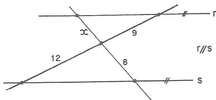
Figura 41 – Aplicando o Teorema de Tales em atividade 6 através de feixe de retas paralelas. Fonte: (MORGADO; WAGNER; JORGE, 2002).
