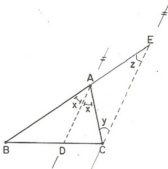
Figura 14 – Demonstrando o Teorema 2.4.
