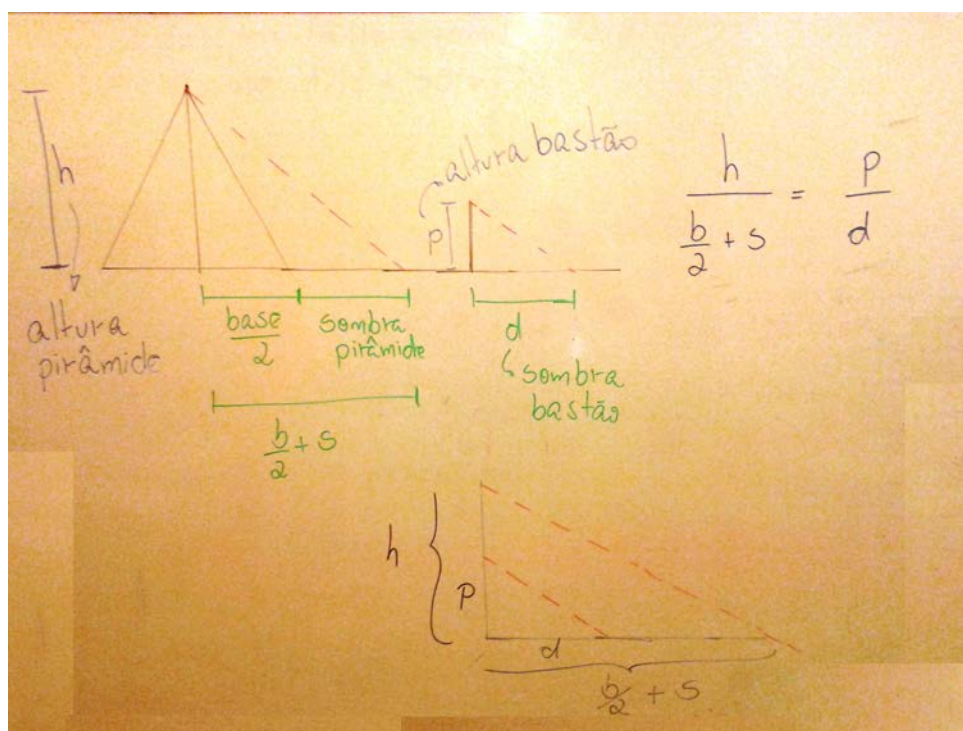
Figura 25 – Representação do cálculo da altura da pirâmide de Quéops.
