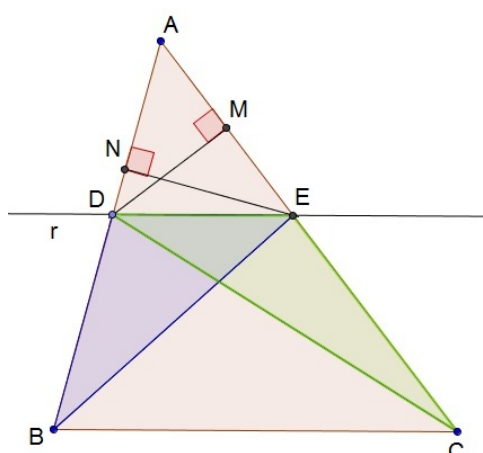
Figura 10 – Demonstrando o Teorema 2.3 usando áreas.
