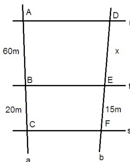
Figura 8 – Aplicando o Teorema 2.2 no Exemplo 2.1.
