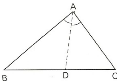
Figura 13 – O Teorema 2.4 (Bissetriz Interna).
