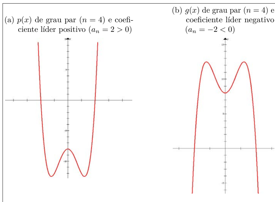
Figura 18 – Registro gráfico das funções polinomiais p(x) = 2(x - 2)(x + 2)(x^2 + 1) e g(x) = -2(x - 2)(x + 2)(x^2 + 1)
