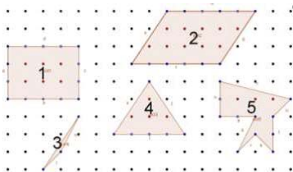
Figura 9 – Polígonos simples
