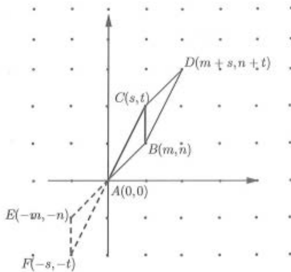
Figura 10 – Paralelogramo fundamental
