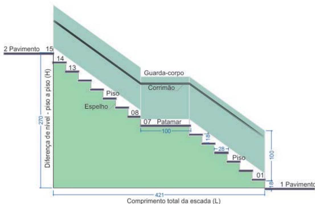
Figura 10 – Textos longos
