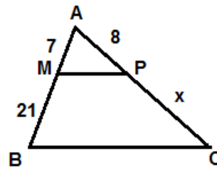
Figura 26 – Exemplo do Teorema e Tales em Triângulos
