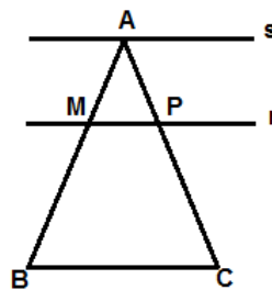
Figura 25 – Teorema de Tales no Triângulo ABC
