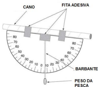
Figura 77 – Teodolito Caseiro
