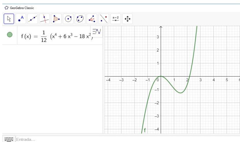
Figura 70 – Gráfico da função f(x) = \frac{1}{12} \cdot (x^4 + 6x^3 - 18x^2)
