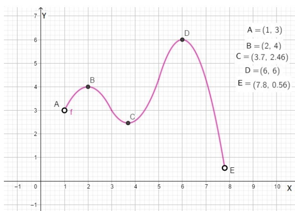
Figura 21 – Máximo e mínimo: Relativo X Absoluto
