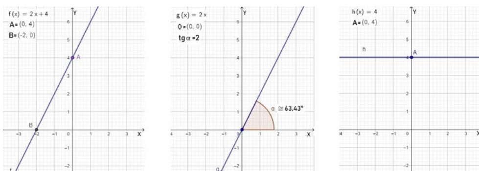
Figura 8 – Gráfico das funções f(x) = 2x + 4 , g(x) = 2x e h(x) = 4
