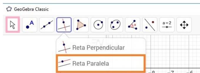
Figura 66 – Explorando o GeoGebra
