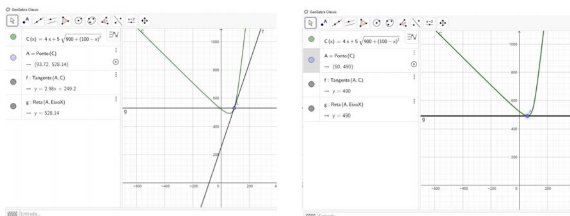
Figura 78 – Encontrando ponto mínimo da função C(x) = 4x + 5\sqrt{30^2 + (100 - x)^2}
