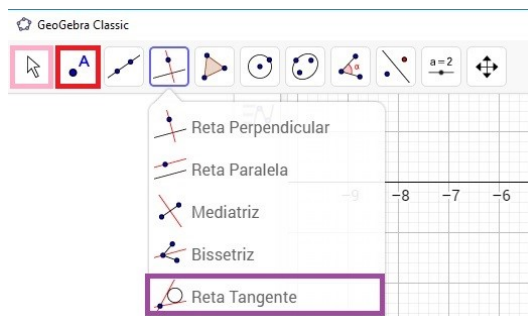
Figura 62 – Explorando a tela inicial do GeoGebra
